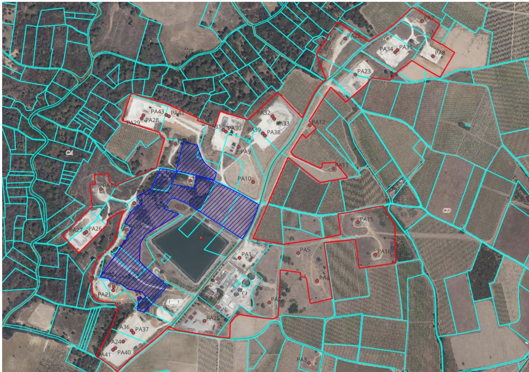
Plan de zonage puits existants et projet d'implantation des nouveaux puits
